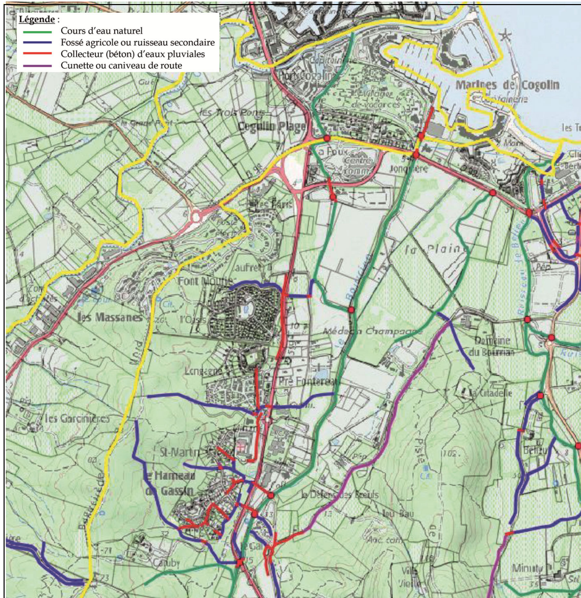
Tracé du réseau pluvial du secteur nord-ouest de la commune (source : AquaConseil, 2018)
