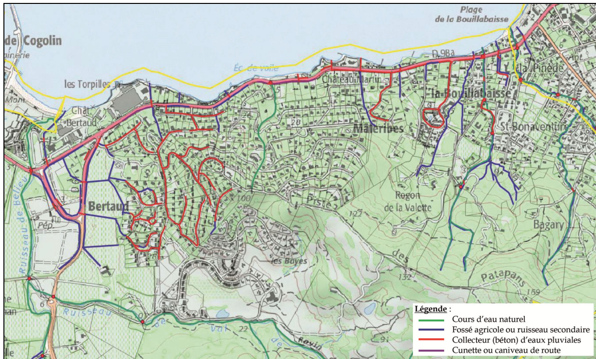
Tracé du réseau pluvial des quartiers côtiers (source : AquaConseil, 2018)
