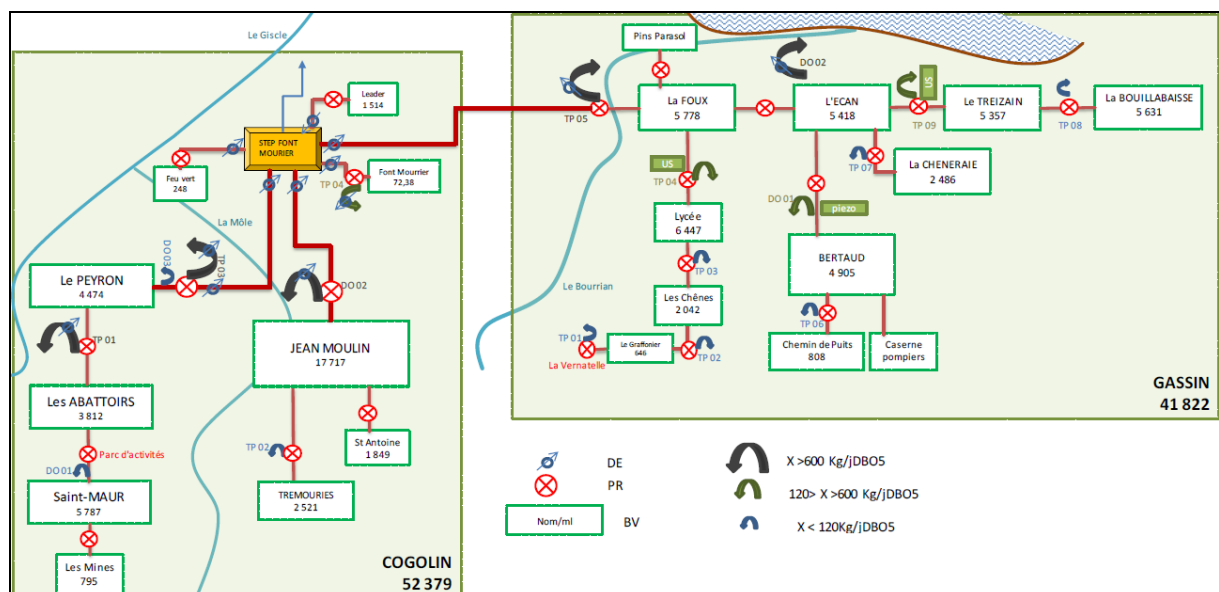
Le synoptique du réseau (source : CCGST 2020)
