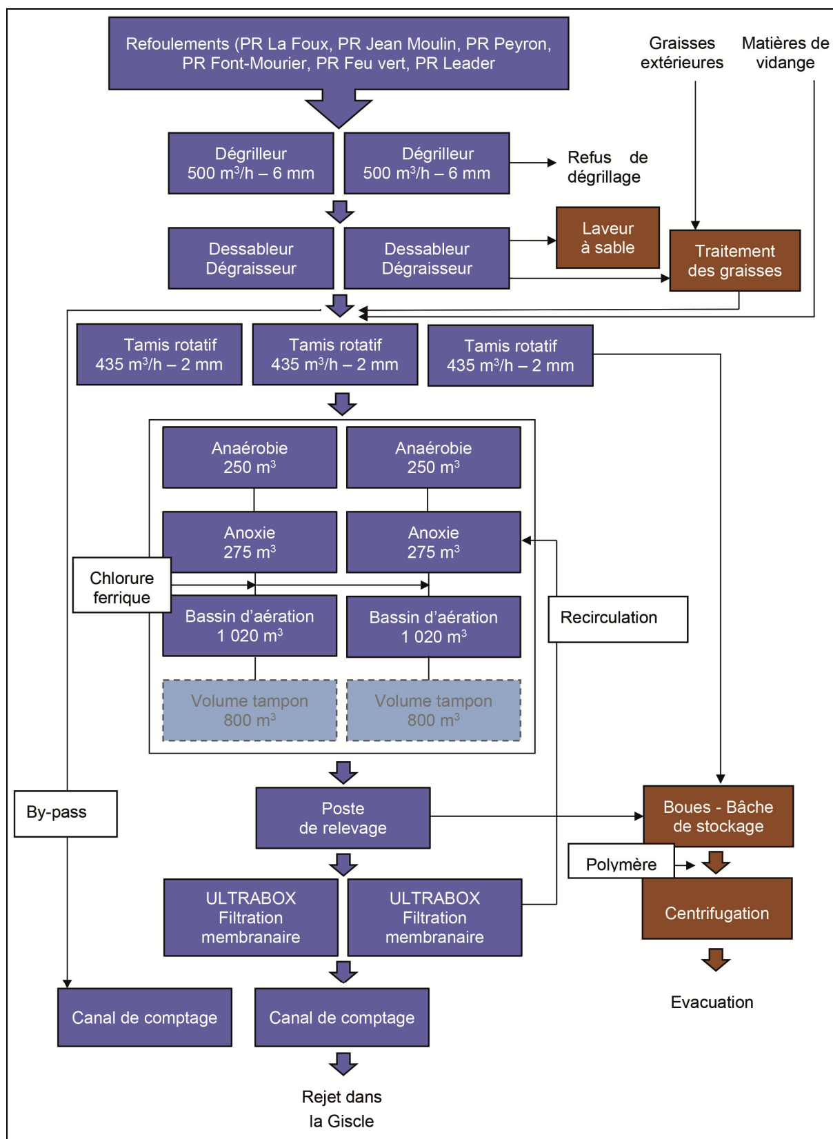
Le synoptique de la station (source : CCGST 2020)
