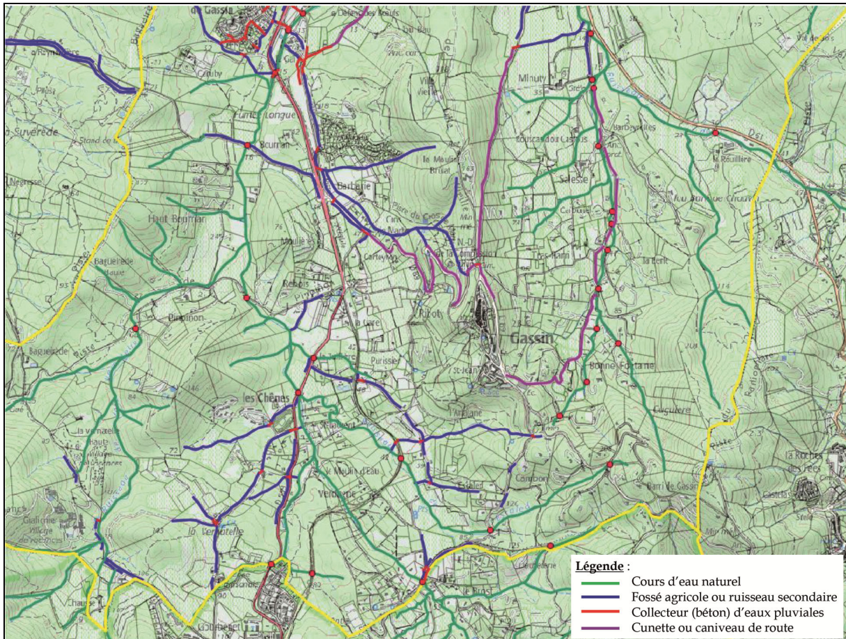
Tracé du réseau pluvial du secteur sud de la commune (source : AquaConseil, 2018)
